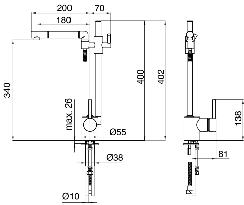
Art. 5500 Miscelatore lavello Sink mixer Mitigeur évier Einhebel - Spültischarmatur
